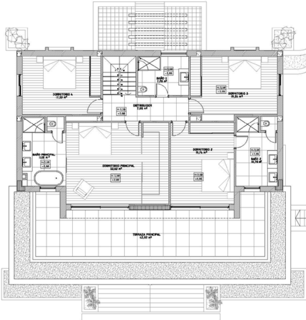
PLANTA ALTA
