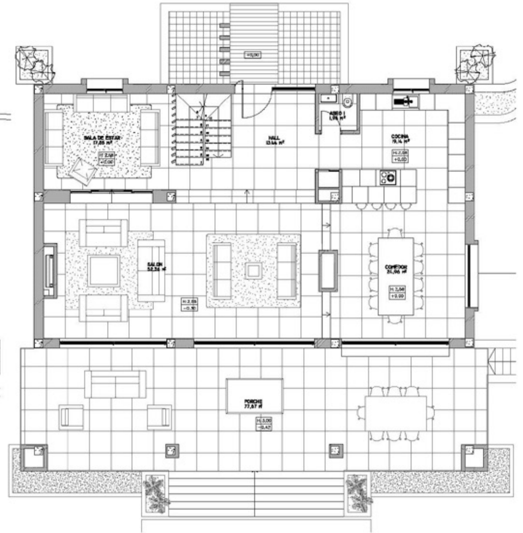
PLANTA BAJA
